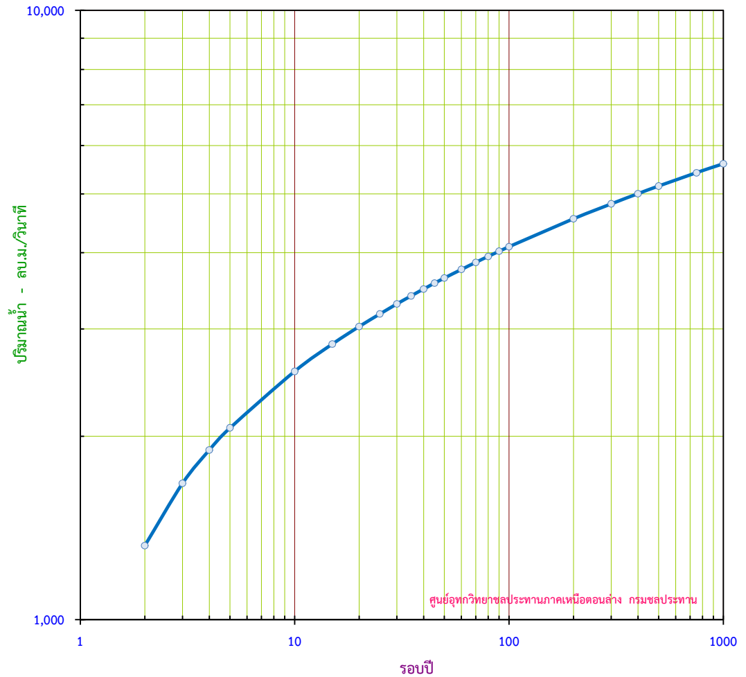
กราฟแสดง ปริมาณน้ำสูงสุดรายปี ขนาดรอบปีต่างๆ สถานี P.15 อ.คลองขลุง จ.กำแพงเพชร
